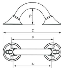
longueur A = taille de la poignée
